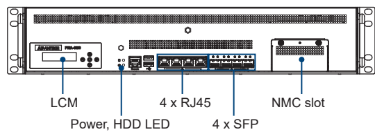
前面板I/O扩展布局图
