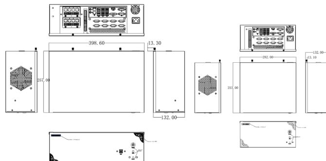
AIMB-Z20机箱
